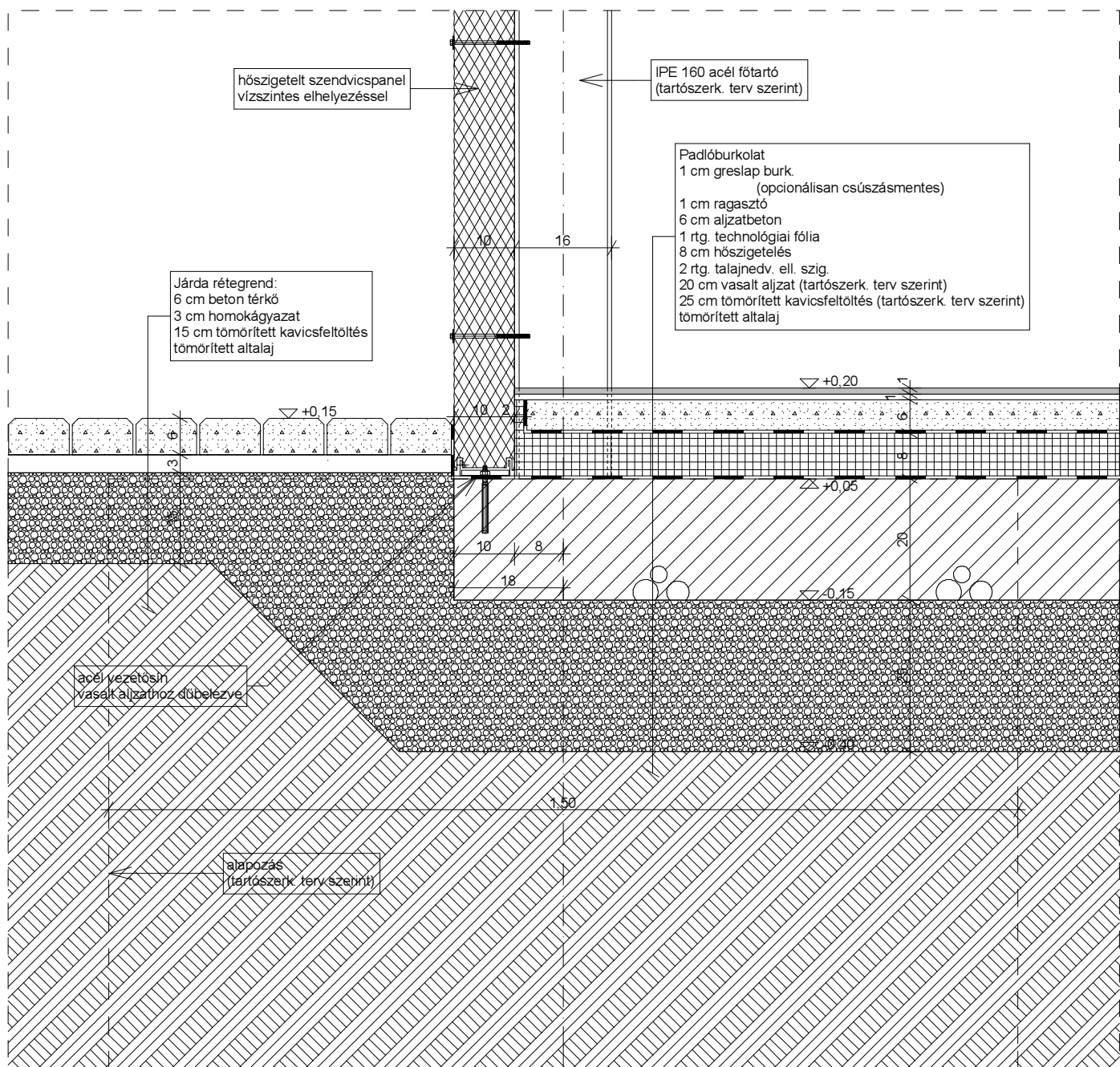
R01 RÉSZLETRAJZ
